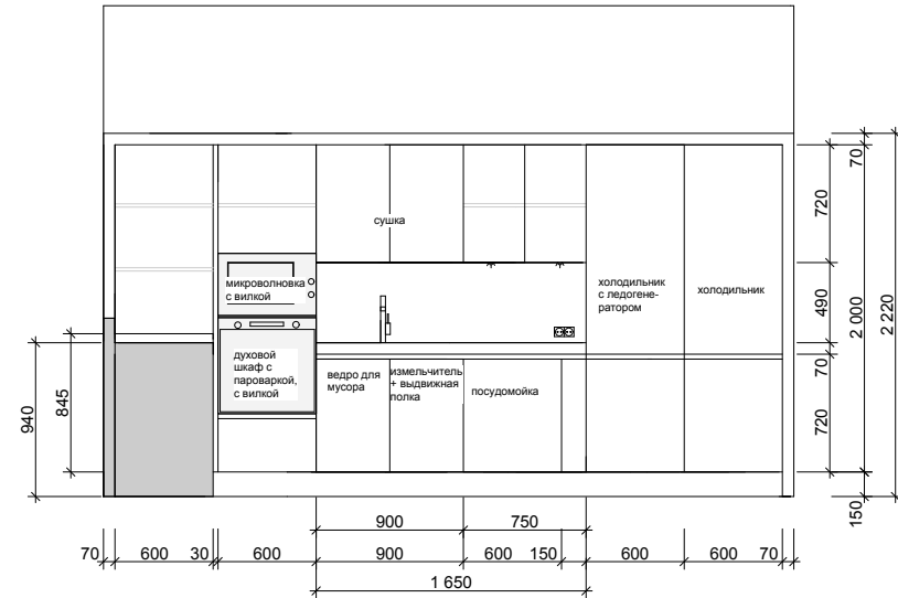
ВИД В
