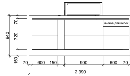
ВИД В
