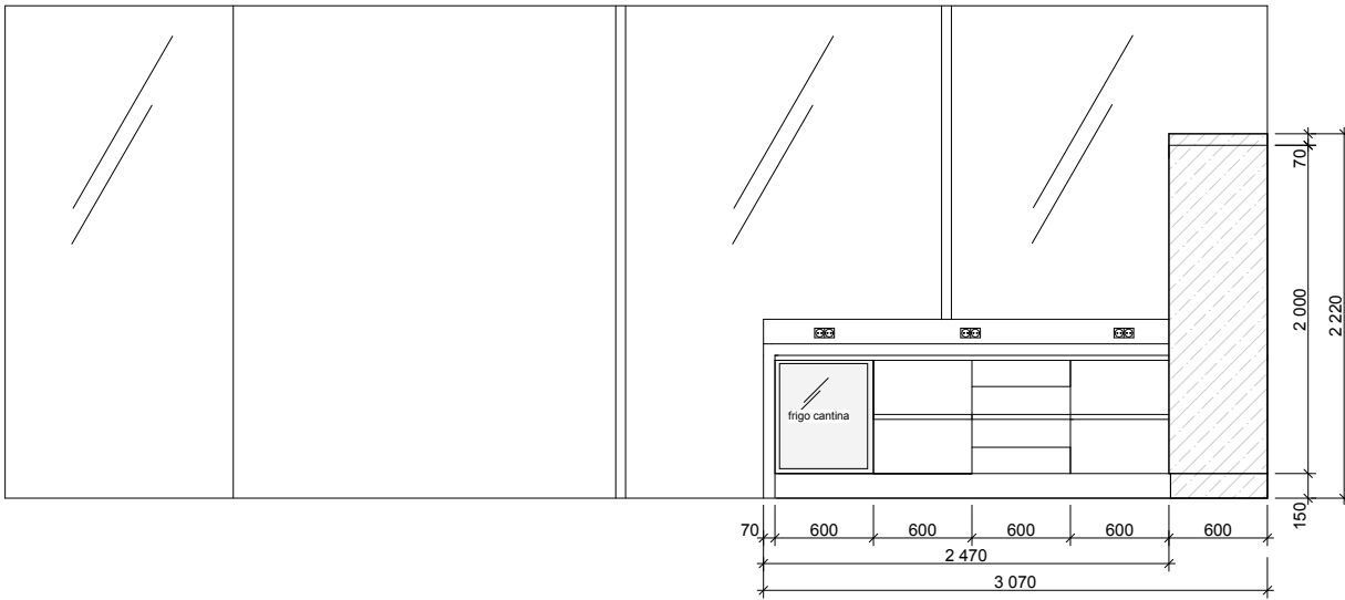
ВИД А
